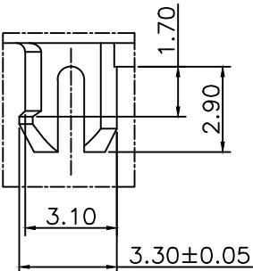
DETAIL A 2:1
